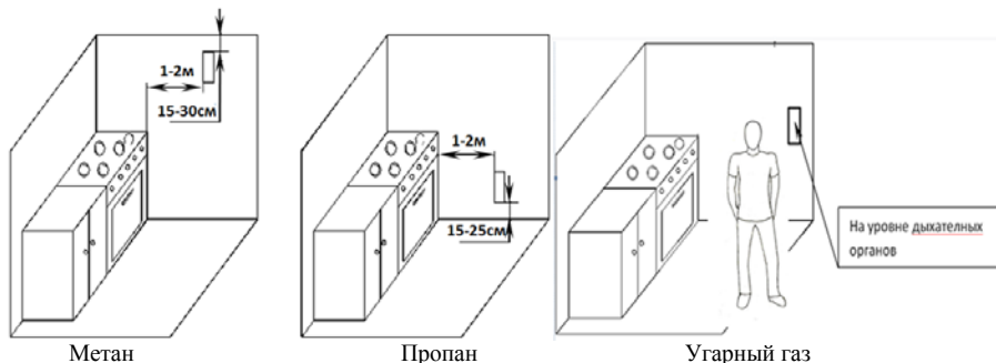
Рисунок 2 – Схема расположения газового сигнализатора
